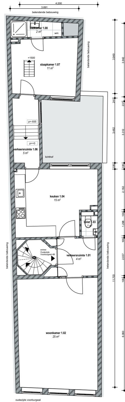
1e verdieping
