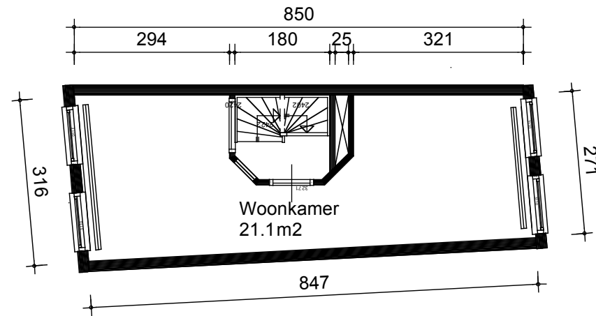
1e verdieping
