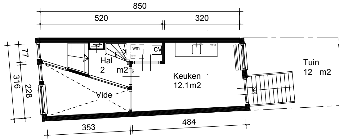
Begane grond / entresol
