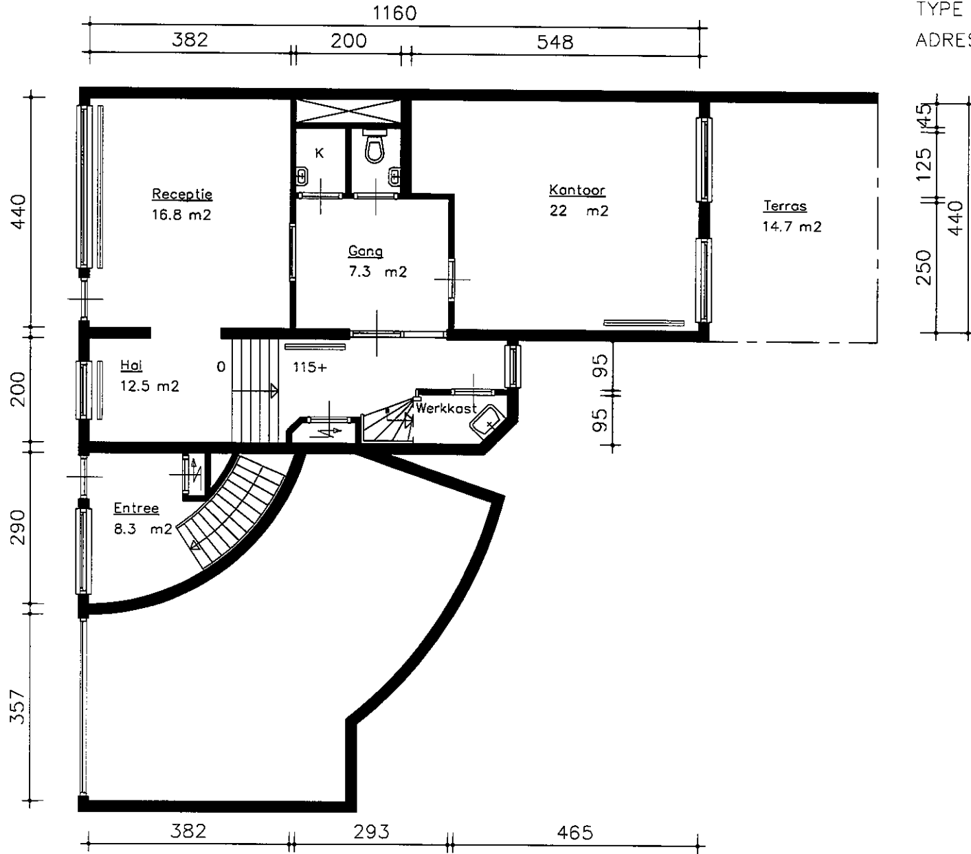
Begane grond
