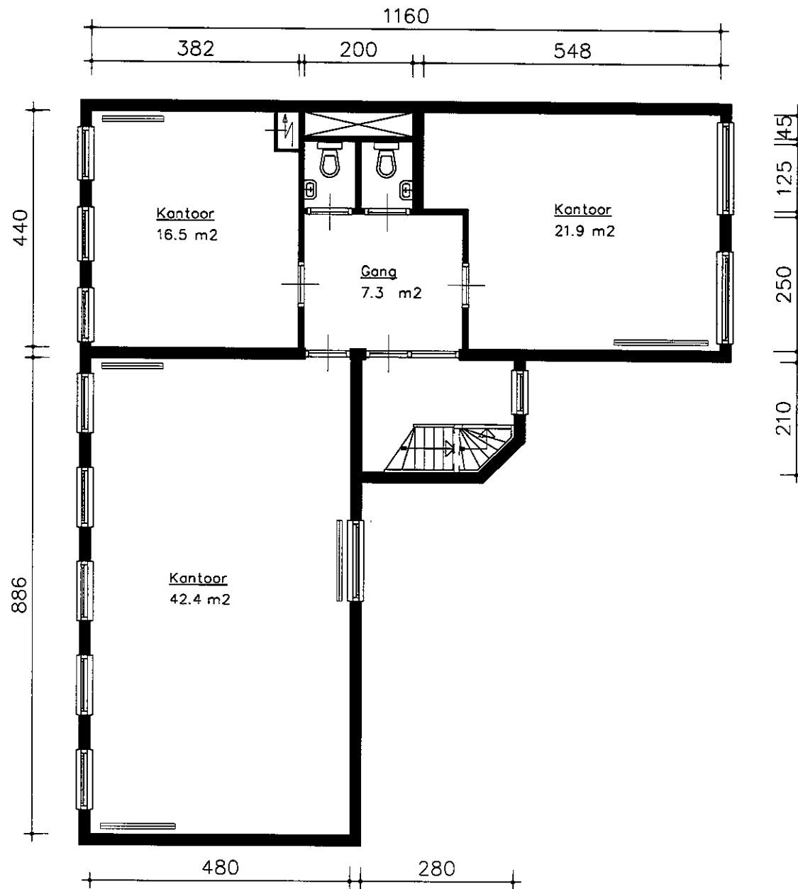
2e verdieping
