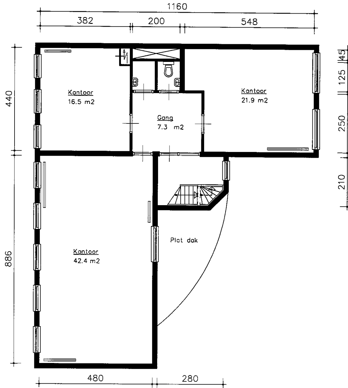
1e verdieping
